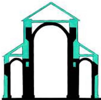
Схема романского храма в разрезе
