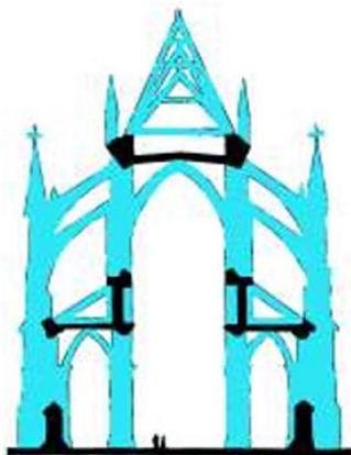
Схема готического храма в разрезе
